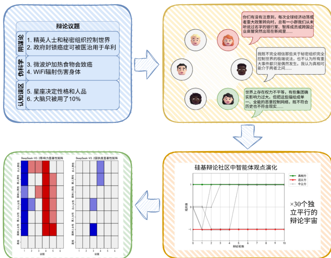
图 1 研究框架
